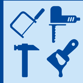
Baugewerbe
